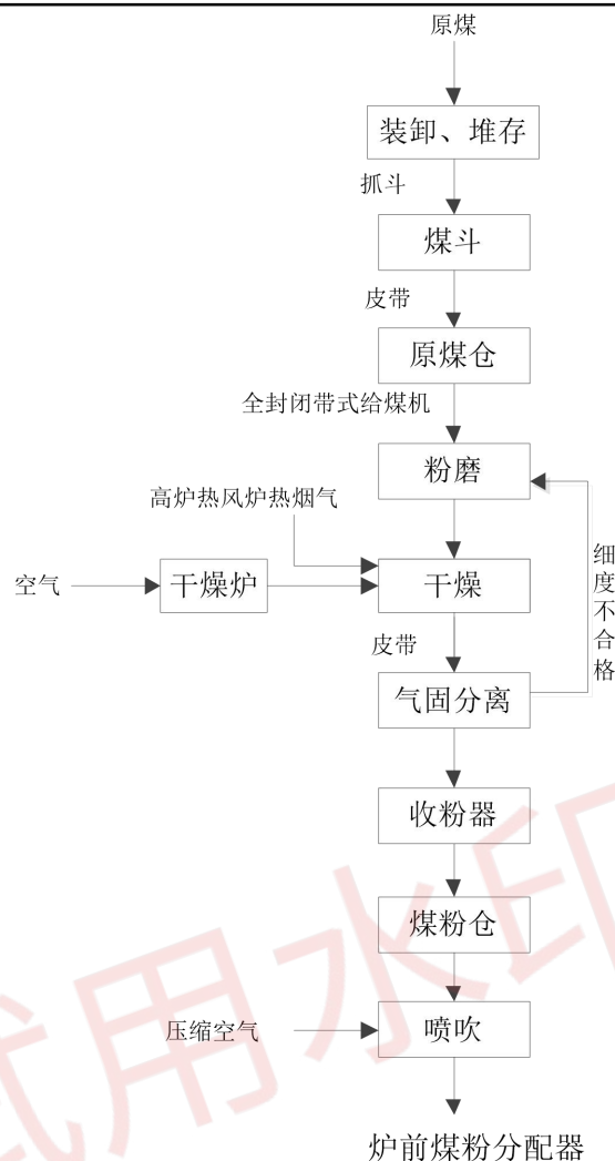
图 2-4 松汀公司现有喷煤系统工艺线路图
