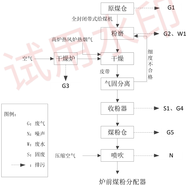
图2-2 工艺流程图及排污位置图
