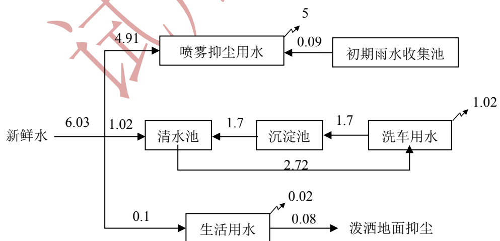
图2-1 项目给排水平衡图
